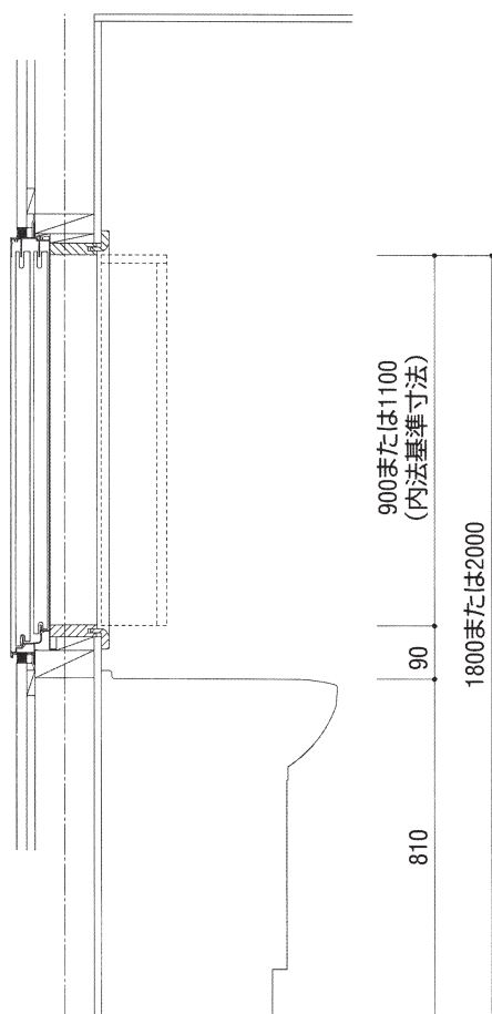
①洗面化粧台を設置する場合
