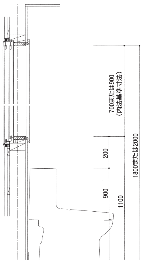
配管スペース（ライニング）がない場合
