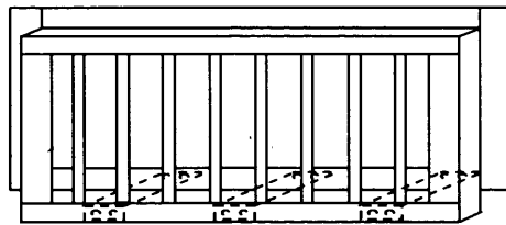
図12-2 面格子をサッシ枠に取付ける場合の構造例
