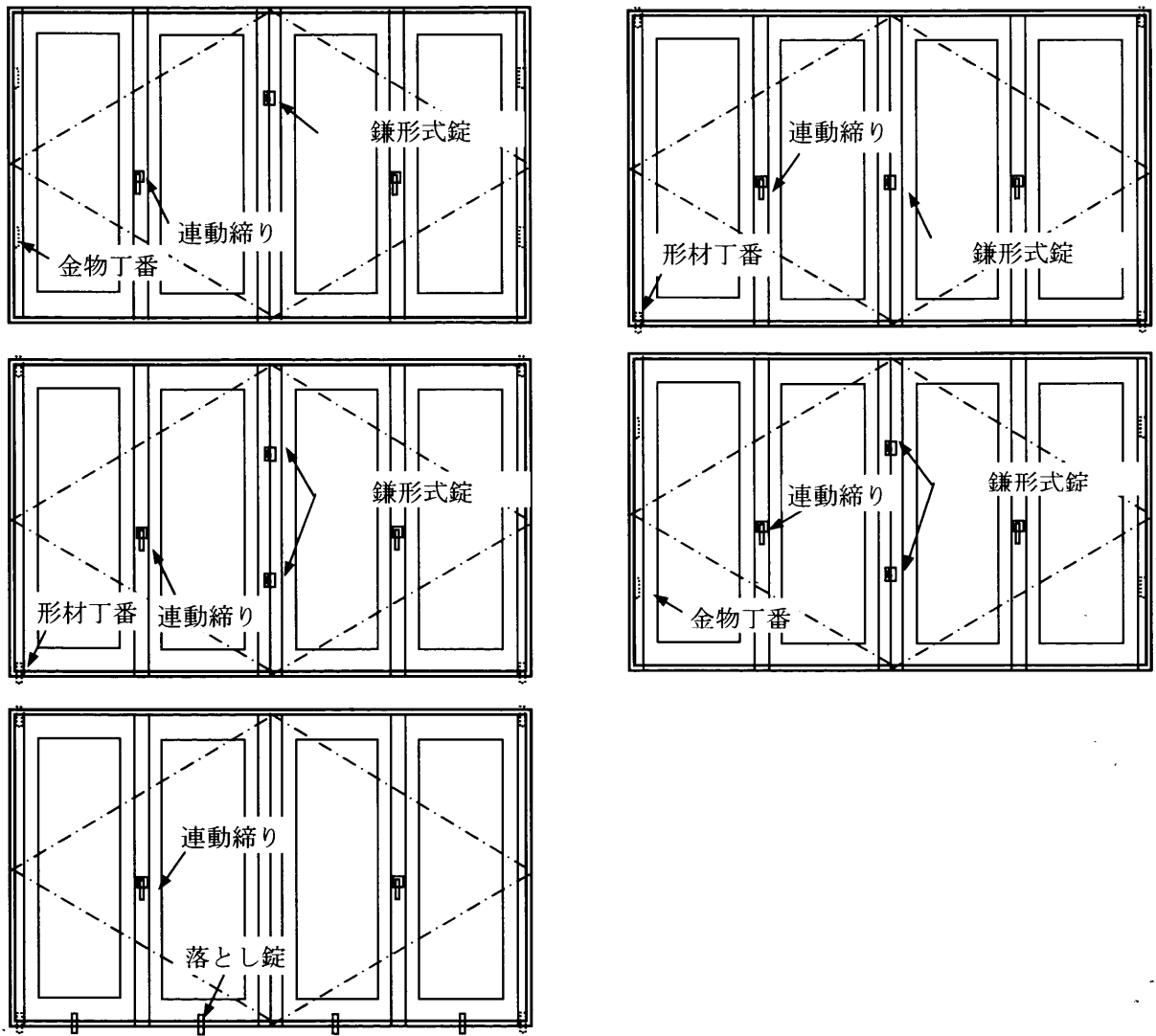
図9 折りたたみ形式のサッシの構造例
