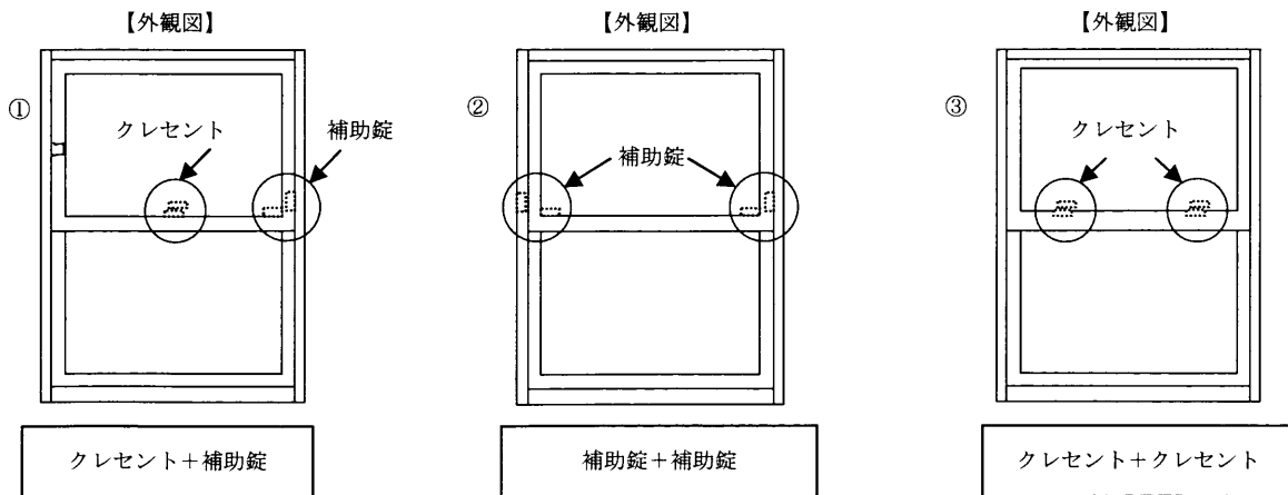
図10 上げ下げ形式のサッシの構造例
