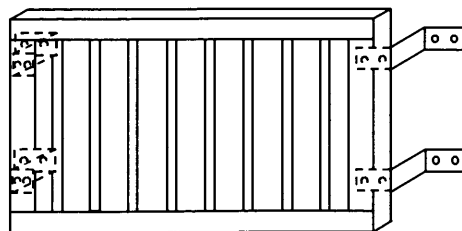
図12-3 面格子を躯体にブラケットにより取付ける場合の構造例
