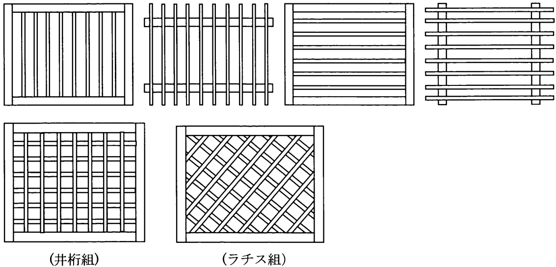
図12-1 面格子 格子組の例
