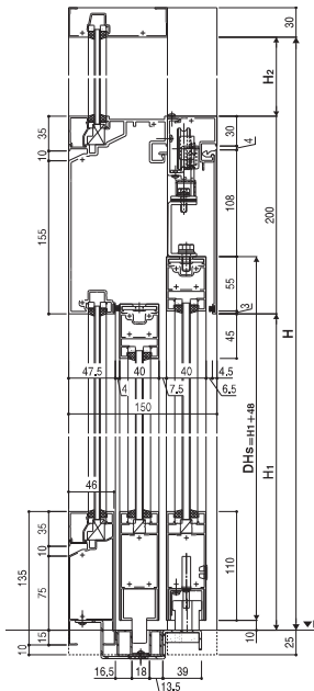
FIX窓 / 防護スクリーン付自動ドア【一般スライド】断面図
