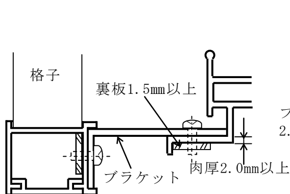
サッシ下枠へのブラケット固定
