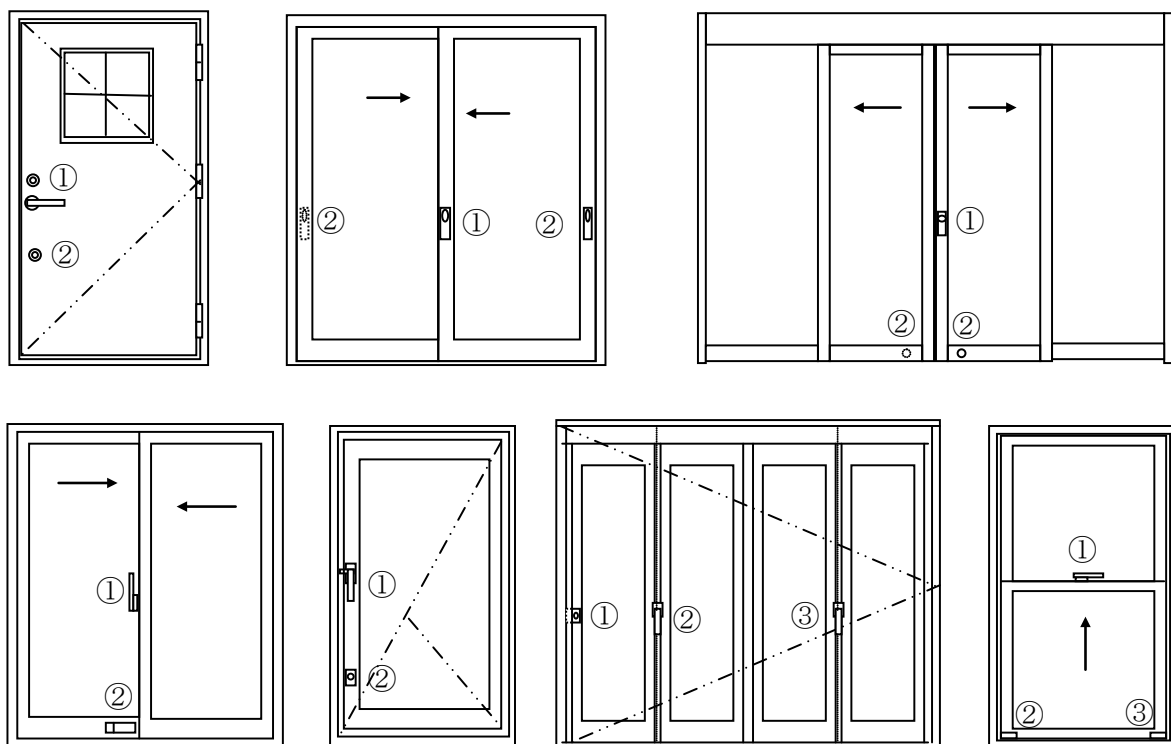
< 2 箇所以上の解錠構造の例 >
