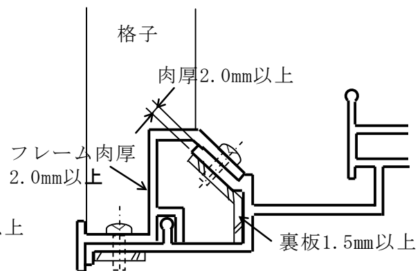
サッシ下枠一体型ブラケット構造
