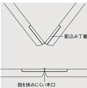
斜めにカットした形状、膨込み丁番で扉と扉の隙間を少なくした*、指挟みにくい木口。
