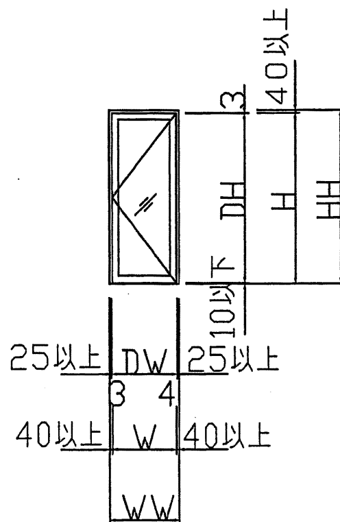
図4 片開き戸の形式
